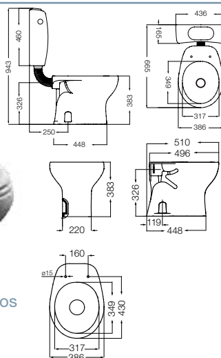
Depósito de colgar una descarga - 6 litros Hanging tank, one flush, 6 liters DME6F B
