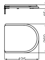
Tapa y asiento inodoro Toilet seat and cover TUX B - herraje plástico / plastic ironwork (HDF) TUXC B / BE / S - herraje metálico / metallic ironwork (MDF) TUR BE / G / S / V - herraje plástico / plastic ironwork (MDF)
