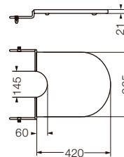
Tapa bidé Cover seat for bidet TRB1U B (1 agujero) / (1 hole) herraje metálico / metallic ironwork (UF) TRB1M B (1 agujero) / (1 hole) herraje metálico / metallic ironwork (MDF)
