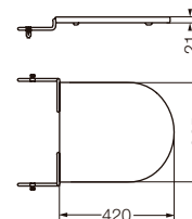
Tapa bidé Cover seat for bidet TRB3U B (3 agujeros) / (3 holes) herraje metálico / metallic ironwork (UF) TRB3M B (3 agujeros) / (3 holes) herraje metálico / metallic ironwork (MDF)
