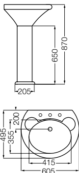
Lavatorio Lavatory LUR1J B / BE / S (1 agujero) / (1 hole) LUR3J B / BE / S (3 agujeros) / (3 holes)
