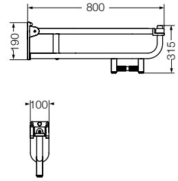
Barral rebatible con portarrollo para accionamiento remoto (no incluye botón, se utiliza el instalado en el depósito) Folding bar with toilet paper holder for remote operation (does not include a button, the one set in the tank is used) VTEPA B
